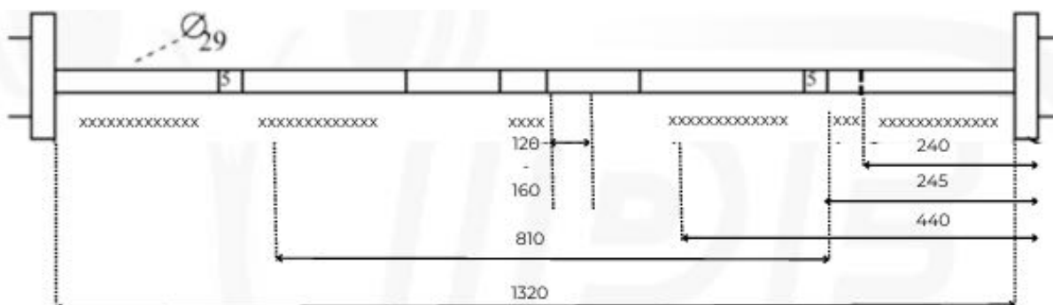
KRAFTLYFTINGASTÖNG SAMÞYKKT AF IPF (ÖLL MÁL Í MM)
